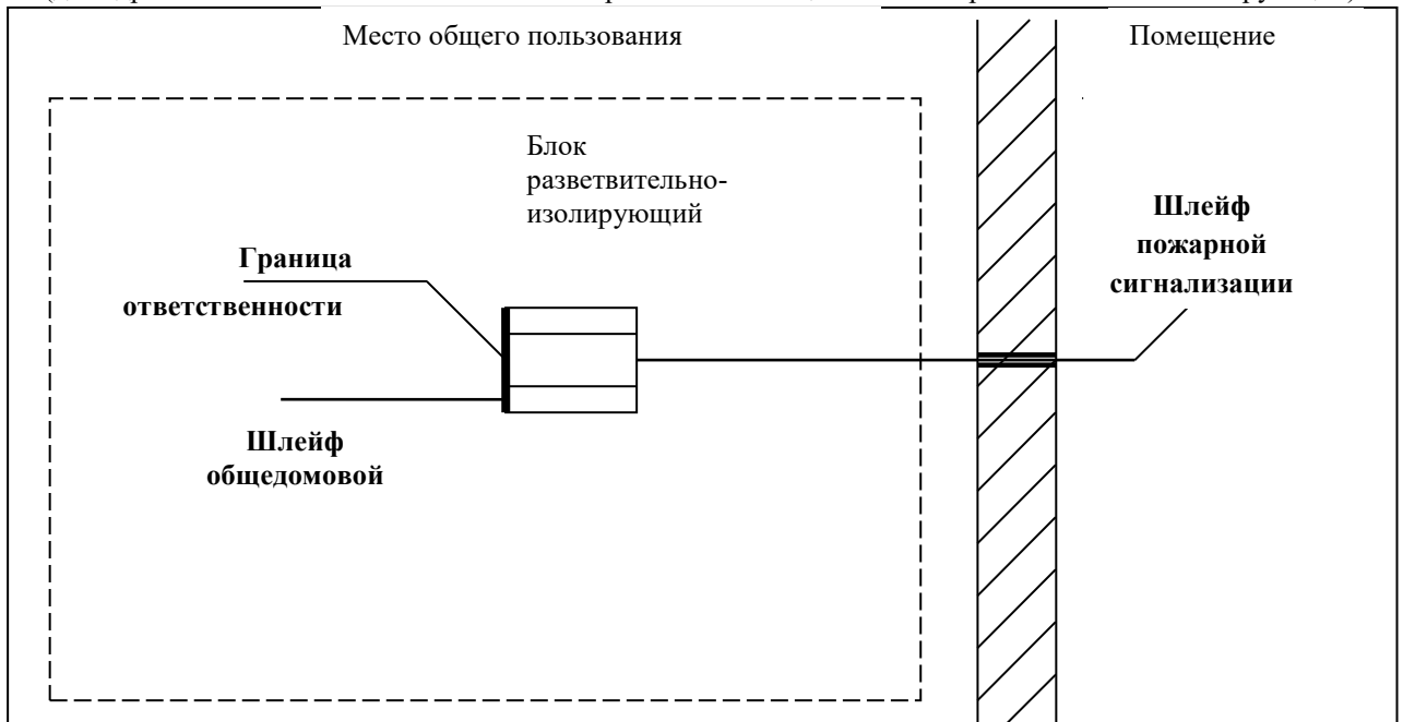
Схема подключения Помещения Владельца (для адресной системы автоматической пожарной сигнализации с блоком разветвительно-изолирующем)
